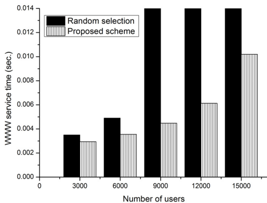
그림 9. 랜덤 선택과 제안방안과의 WWW 서비스 지연시간 (service delay) 비교
