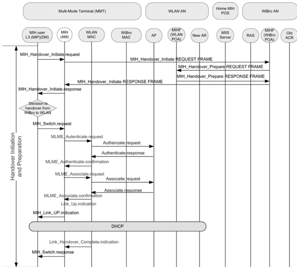
그림 6 WiBro-WLAN Handoff(Handoff initiation and preparation)
