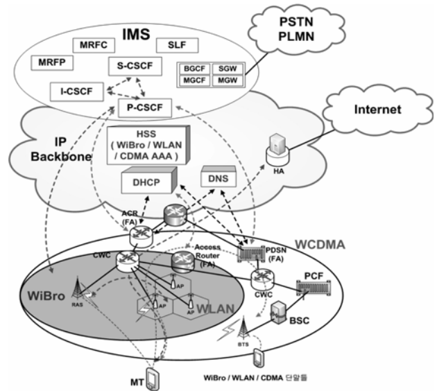
그림 13 MIH를 위한 통합기지국 연동 구조
