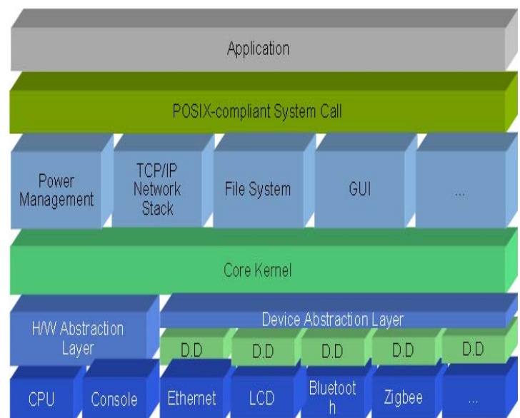
<그림1> KHIX 임베디드 시스템 운영체제 구성도
